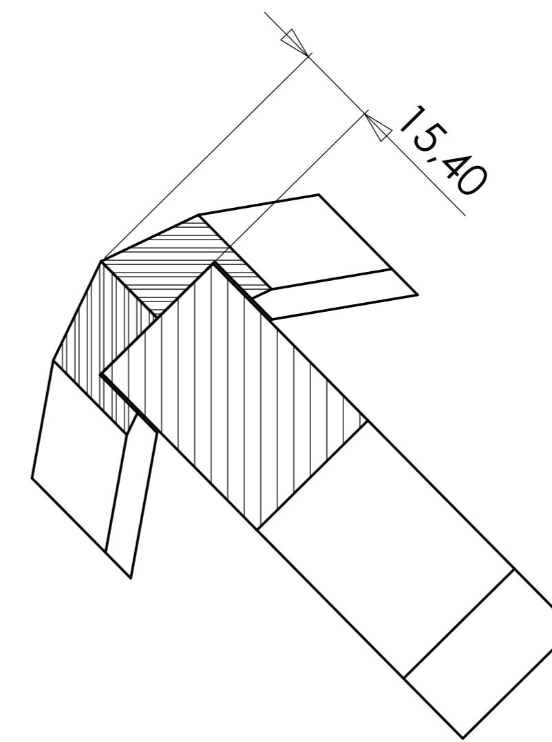
SECTION D-D SCALE 1 : 10
